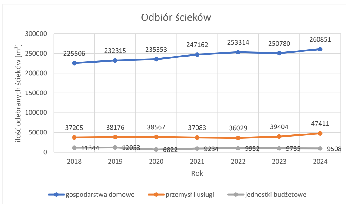
Wykres 3 Odbiór ścieków za 2018-2024
