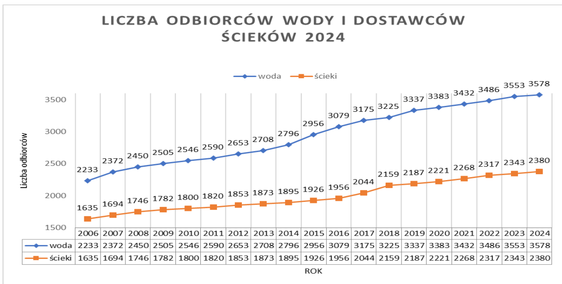
Wykres 5 Liczba odbiorców usług wodociągowych i kanalizacyjnych na koniec roku 2024
